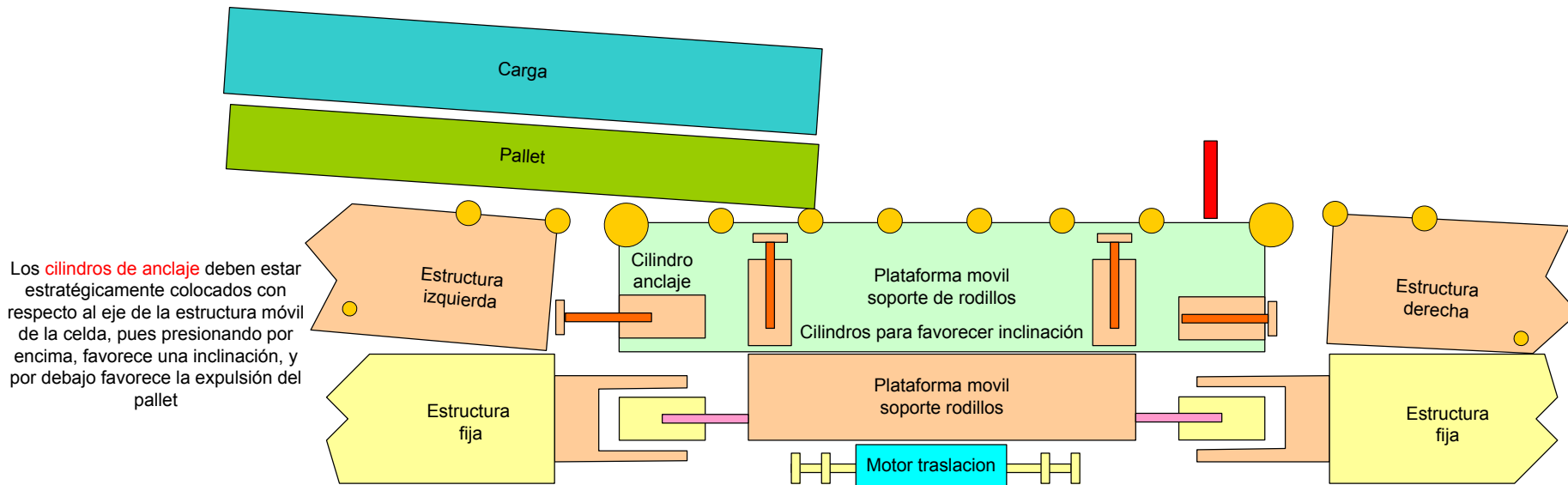
Carro pasando pallet de la celda al carro
