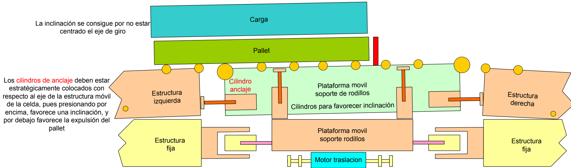
Carro pasando pallet del carro a la celda
